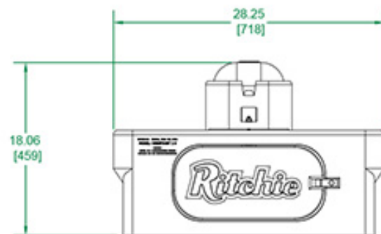
VIEW1 SCALE 1/10
